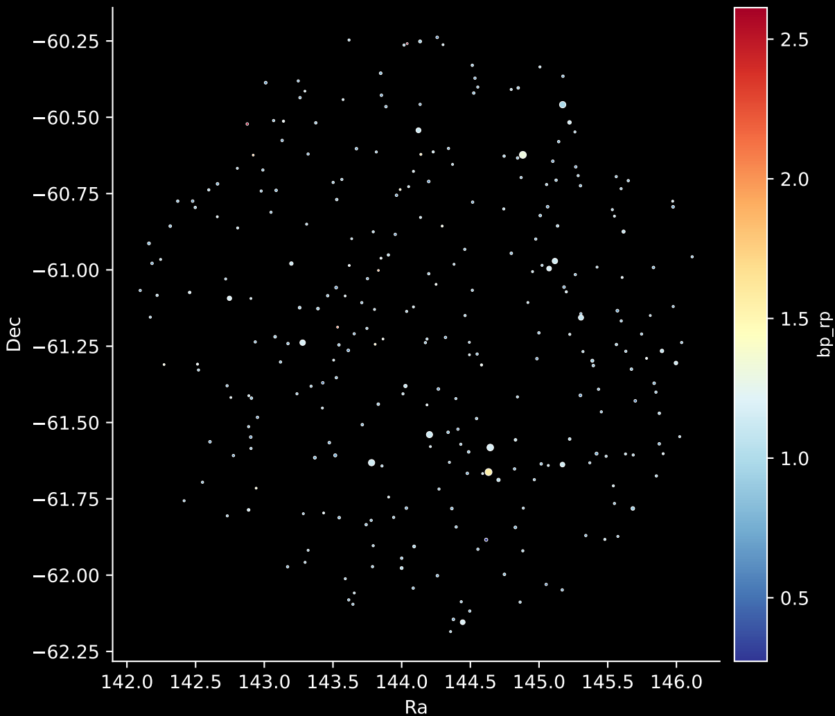
GALAH DR4 Field: [7003] Stars: 293
