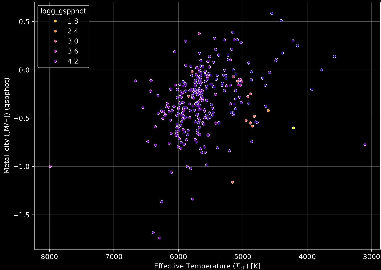
GALAH DR4 Field: [7003] Stellar Population Parameters (n= 293)
