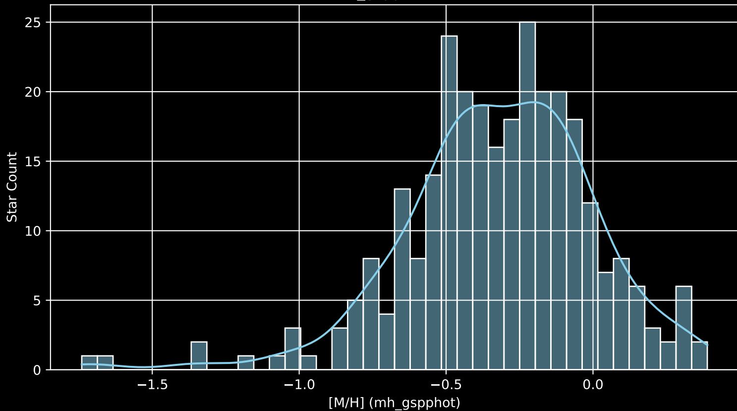
GALAH DR4 Field: [7003] [M/H] (mh_gspphot) (n= 291)
